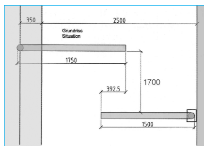
Situationsplan zur Ausführung
