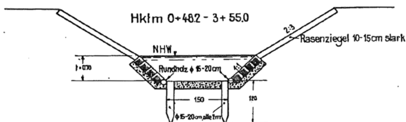
Profil des Vorflutgrabens
